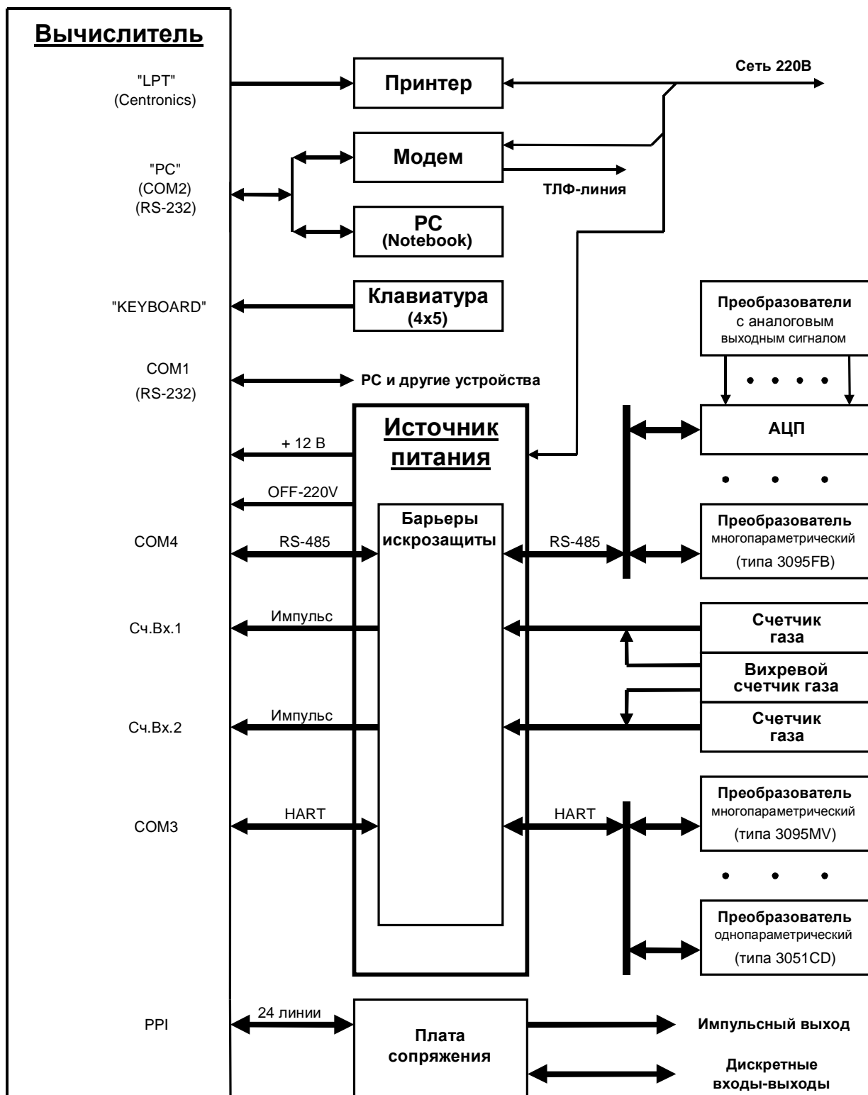
Рисунок А.1. - Схема структурная комплекса на базе вычислителя
